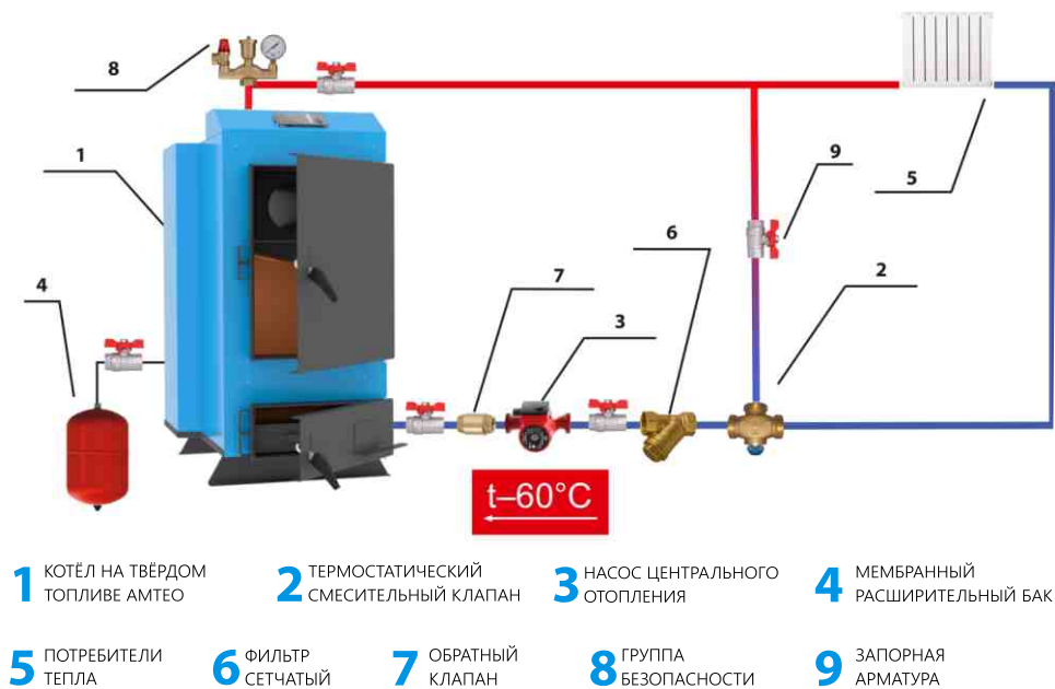
Рисунок 2(а). Типовая схема обвязки котла Amteo с 3-х ходовым клапаном
